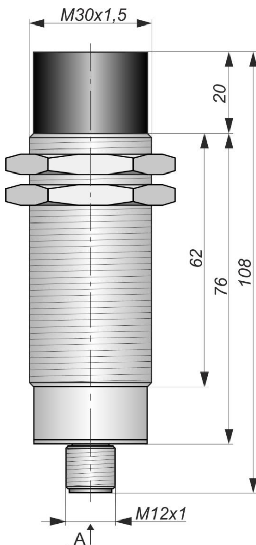
Габаритный чертеж
